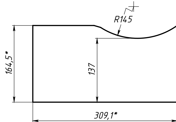
Поз.2 (Угольник)
